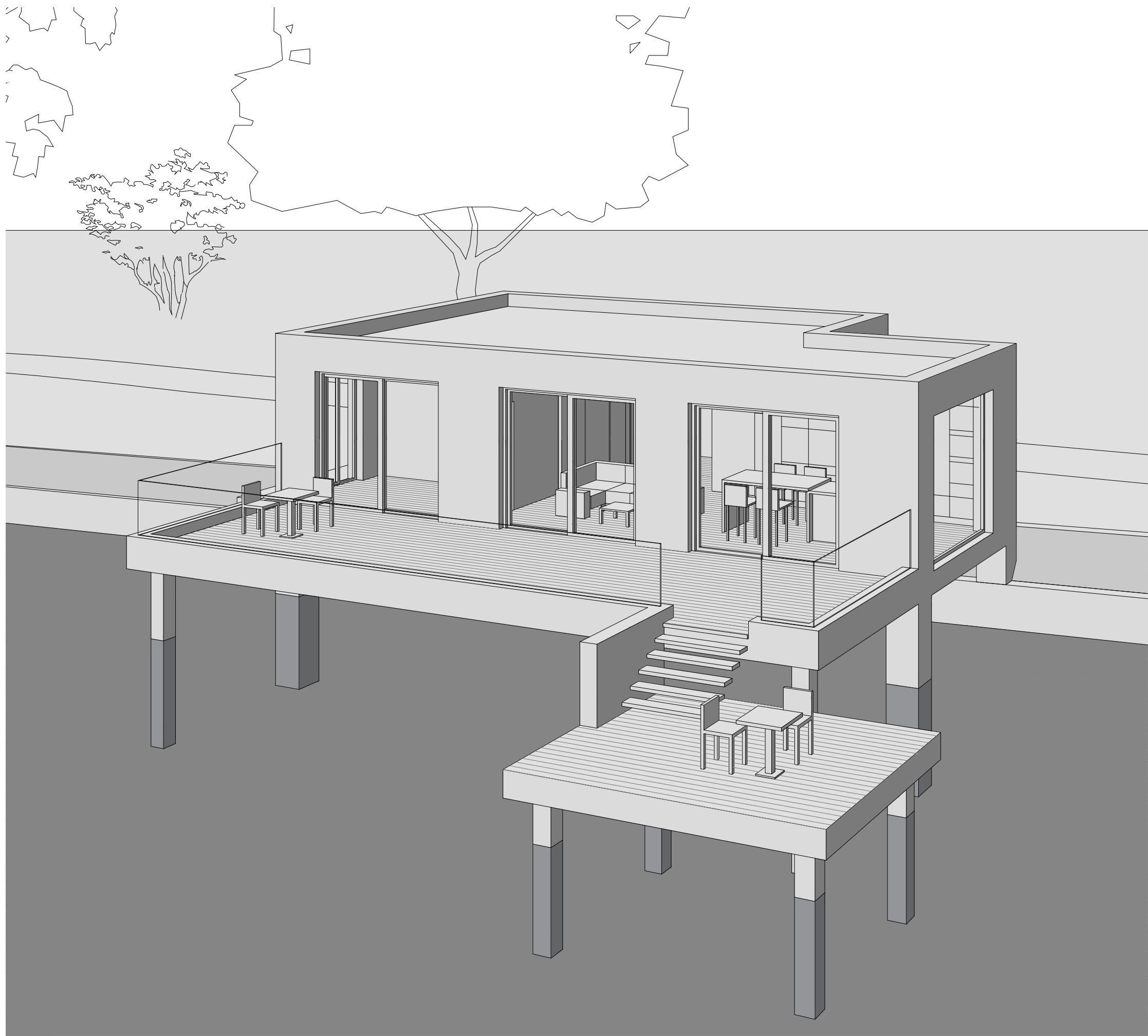
Tweepuntsperspectief (ooghoogte 9m) - zuidwestgevel / AutoCAD
