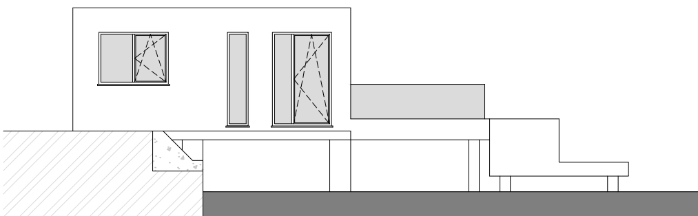
Noordgevel / AutoCAD
