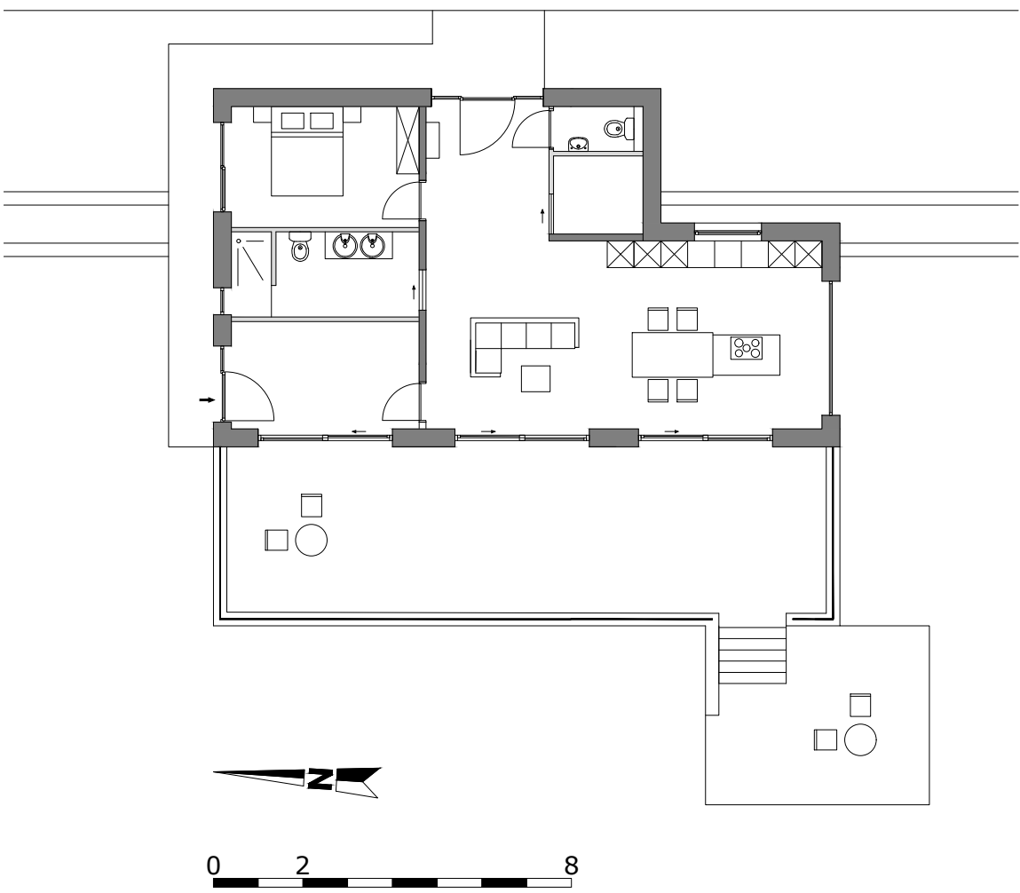
Gelijkvloers / AutoCAD
