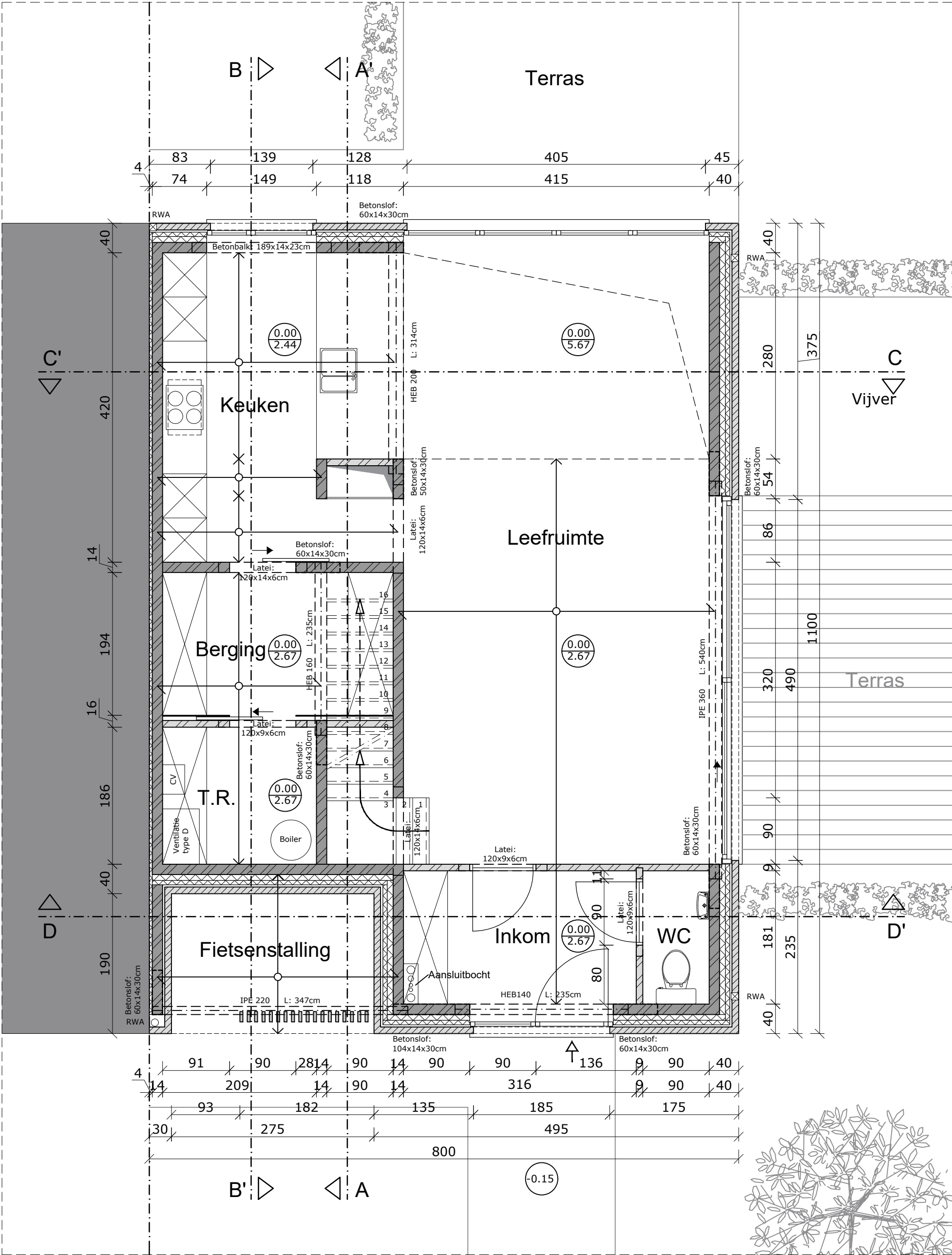
Gelijkvloers
