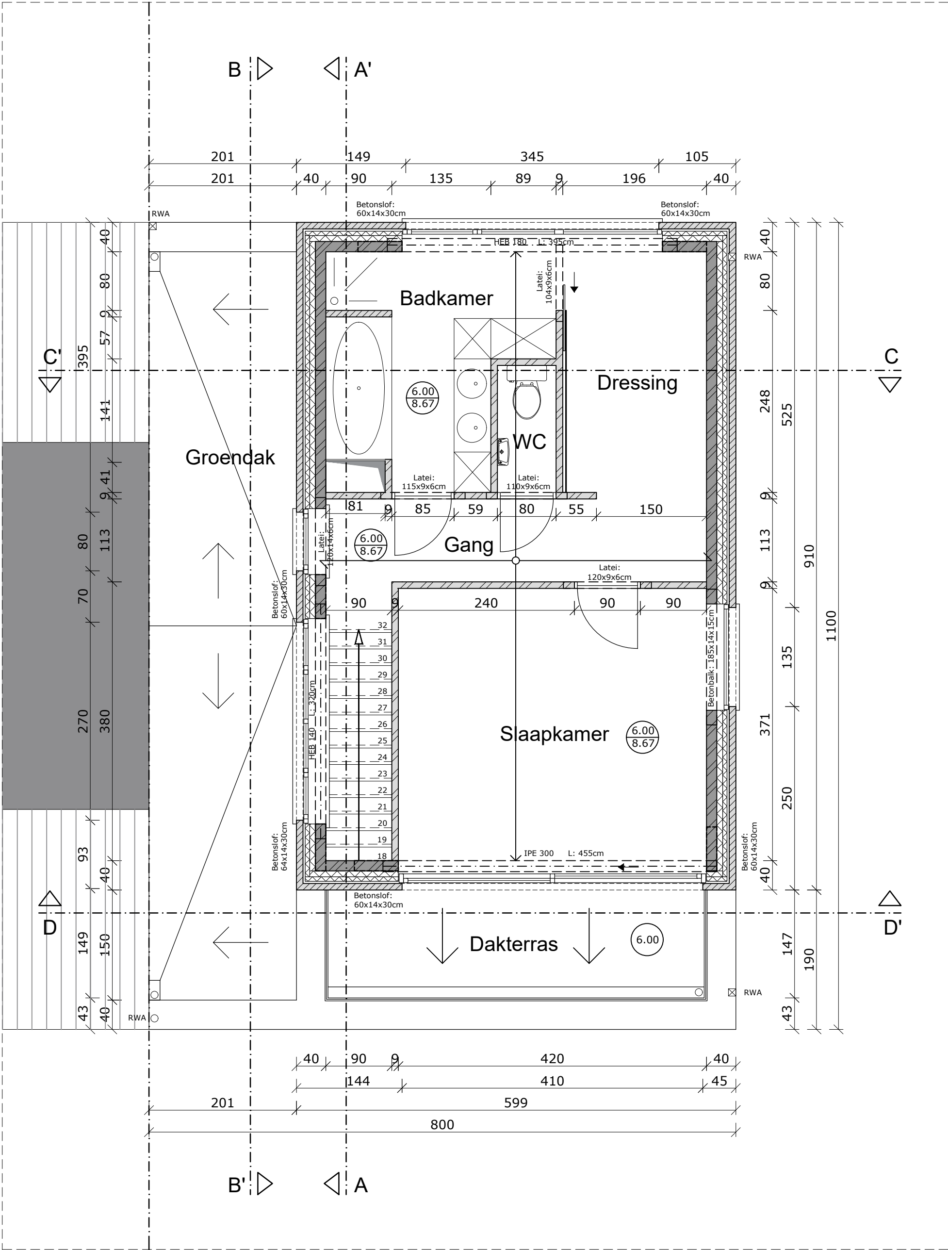
2de verdieping
