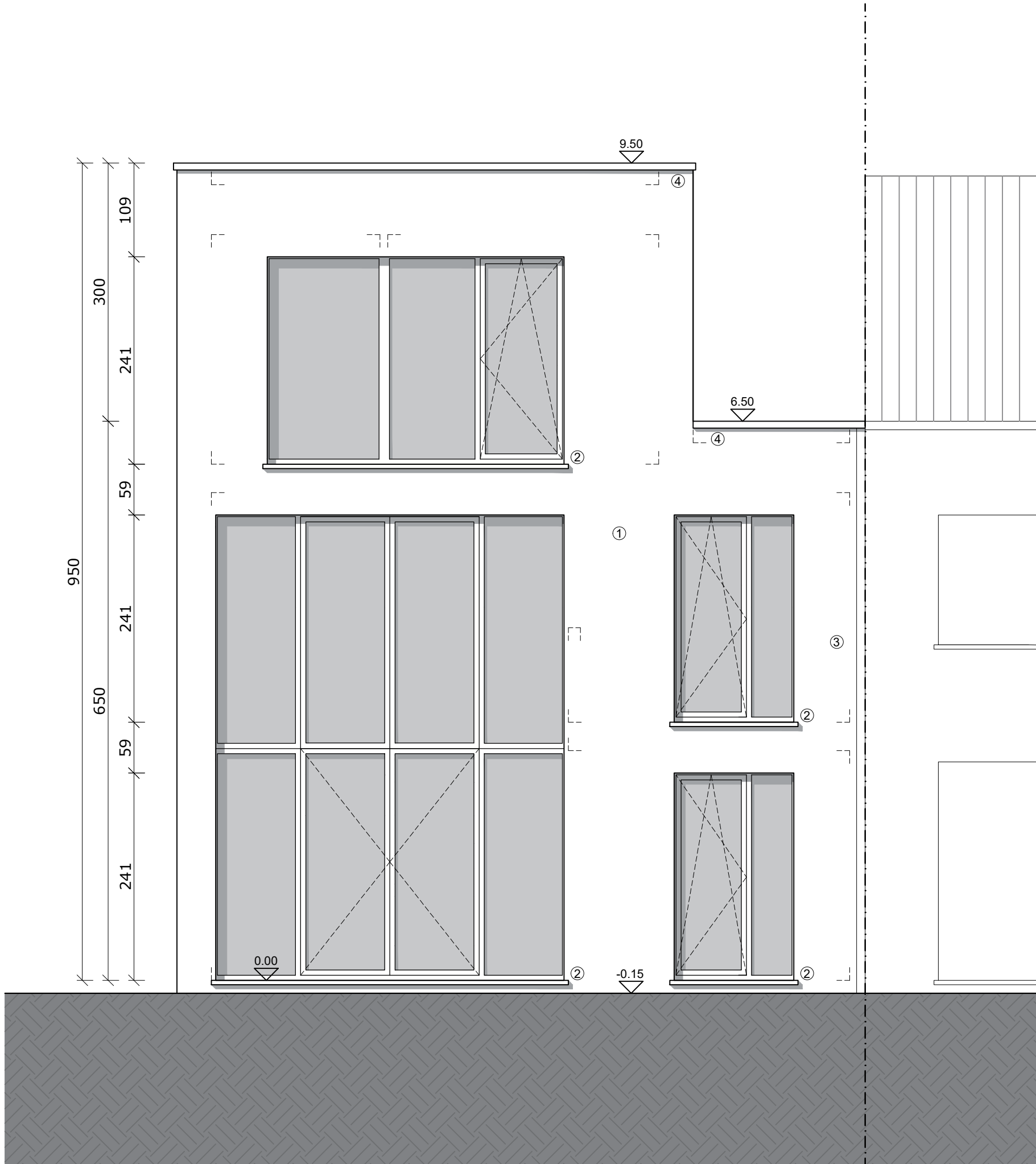
Achtergevel (westen)
