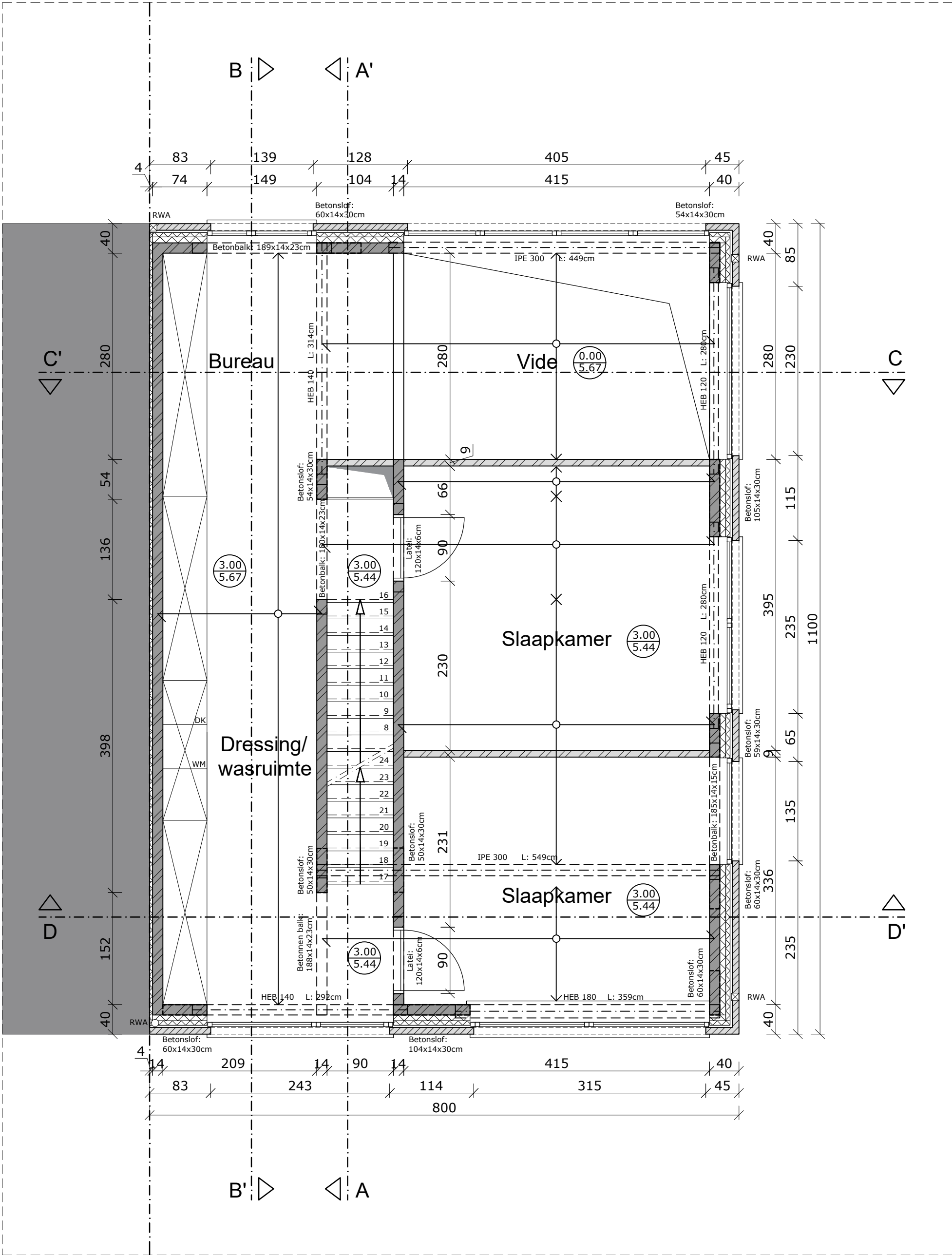
1ste verdieping
