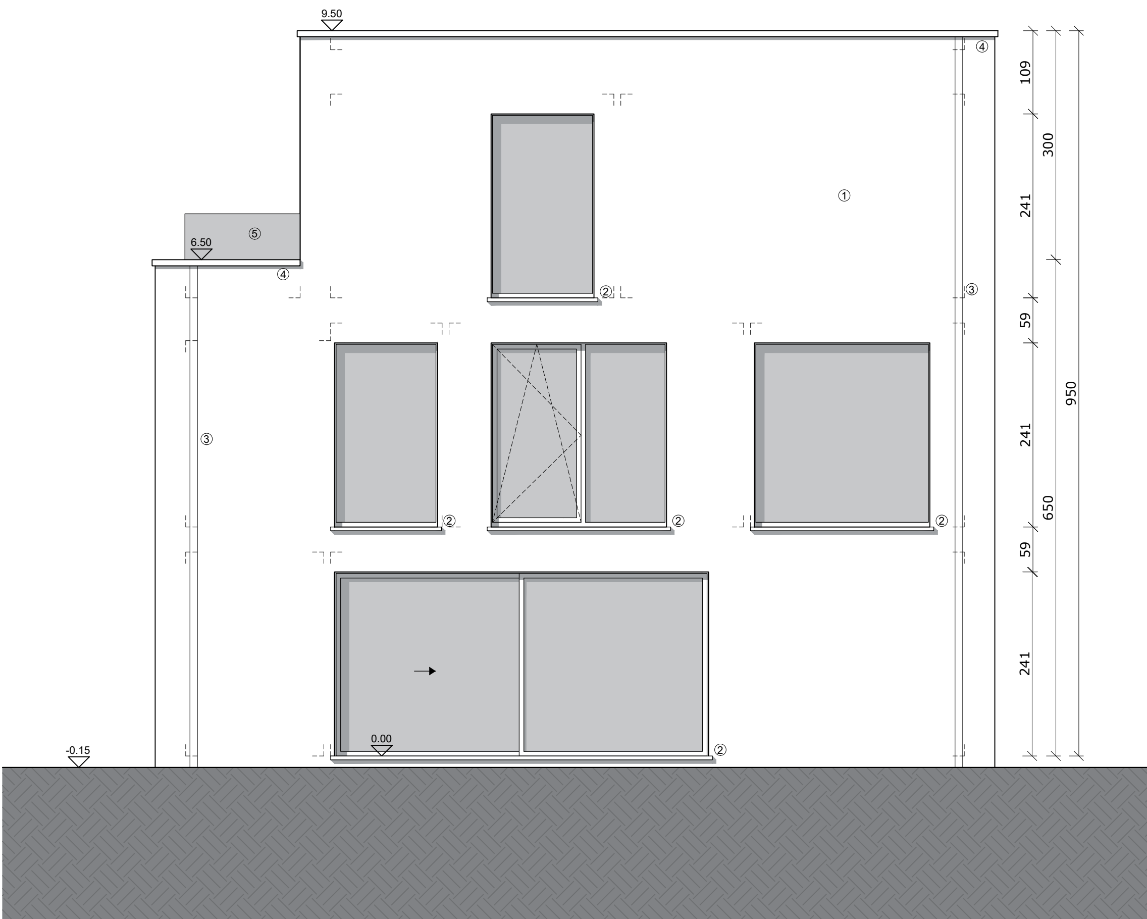
Zijgevel (noorden)
