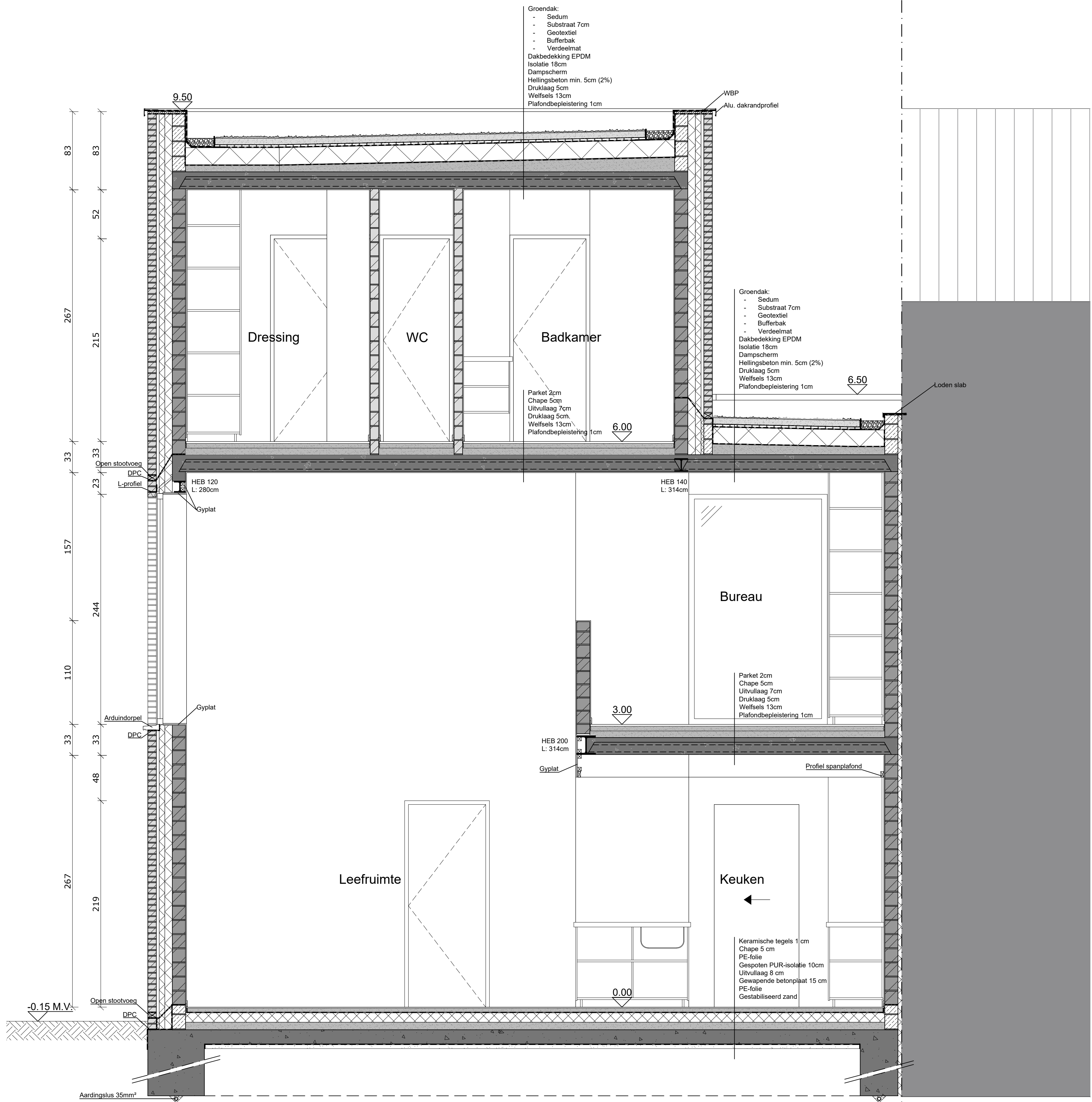
Doorsnede CC'
