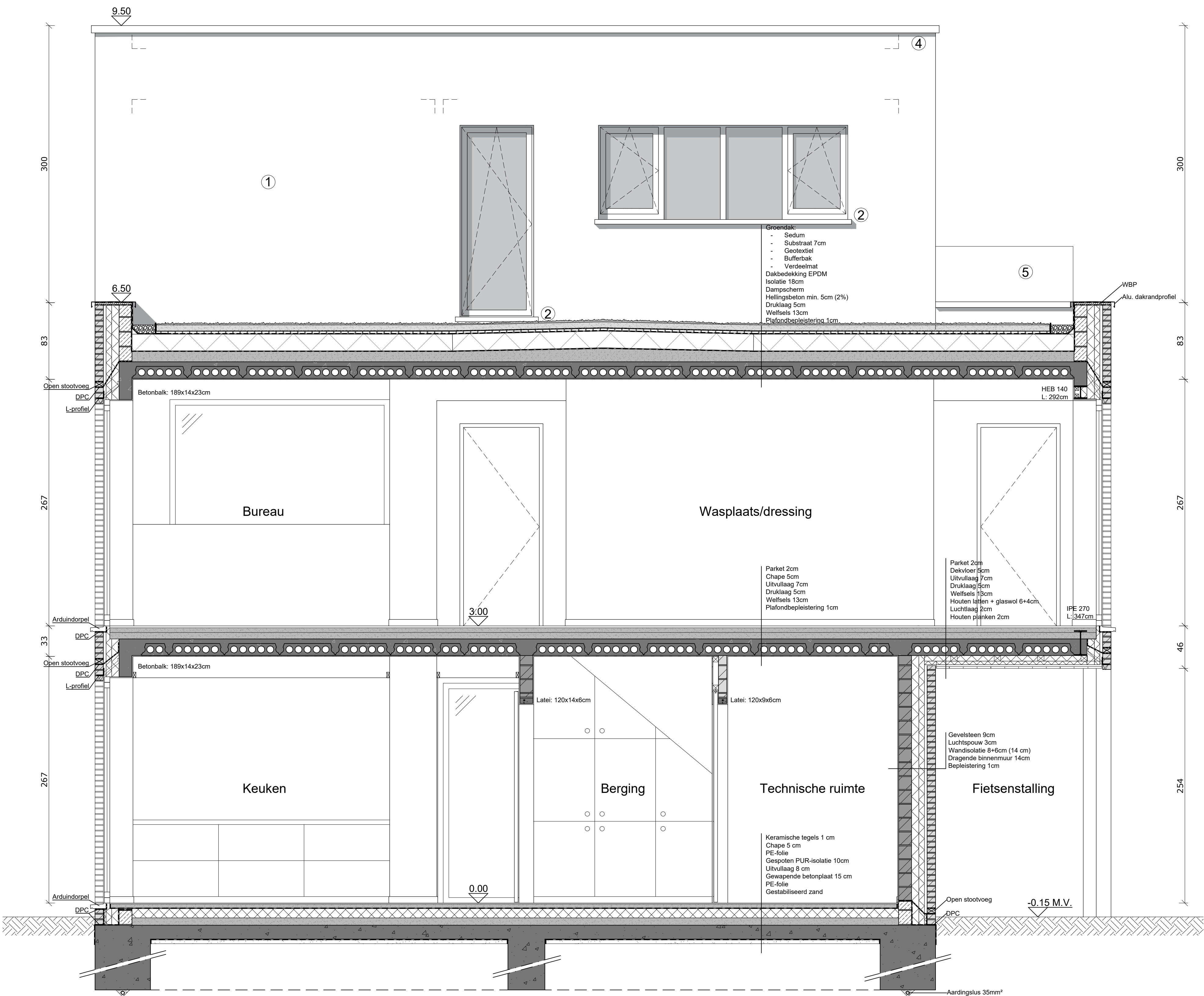
Doorsnede BB'
