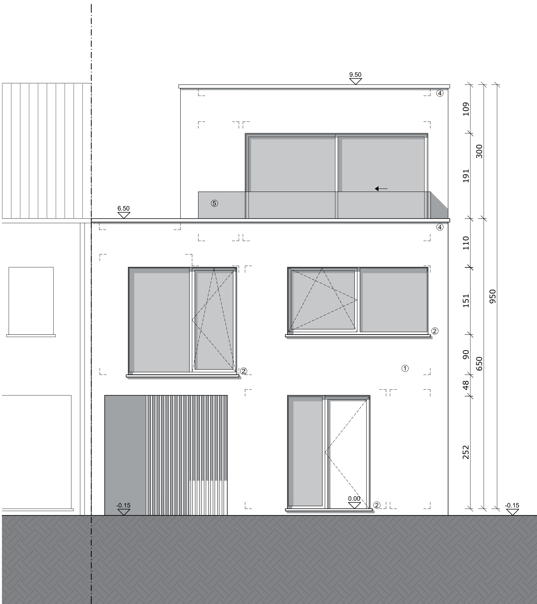
Voorgevel (oosten)
