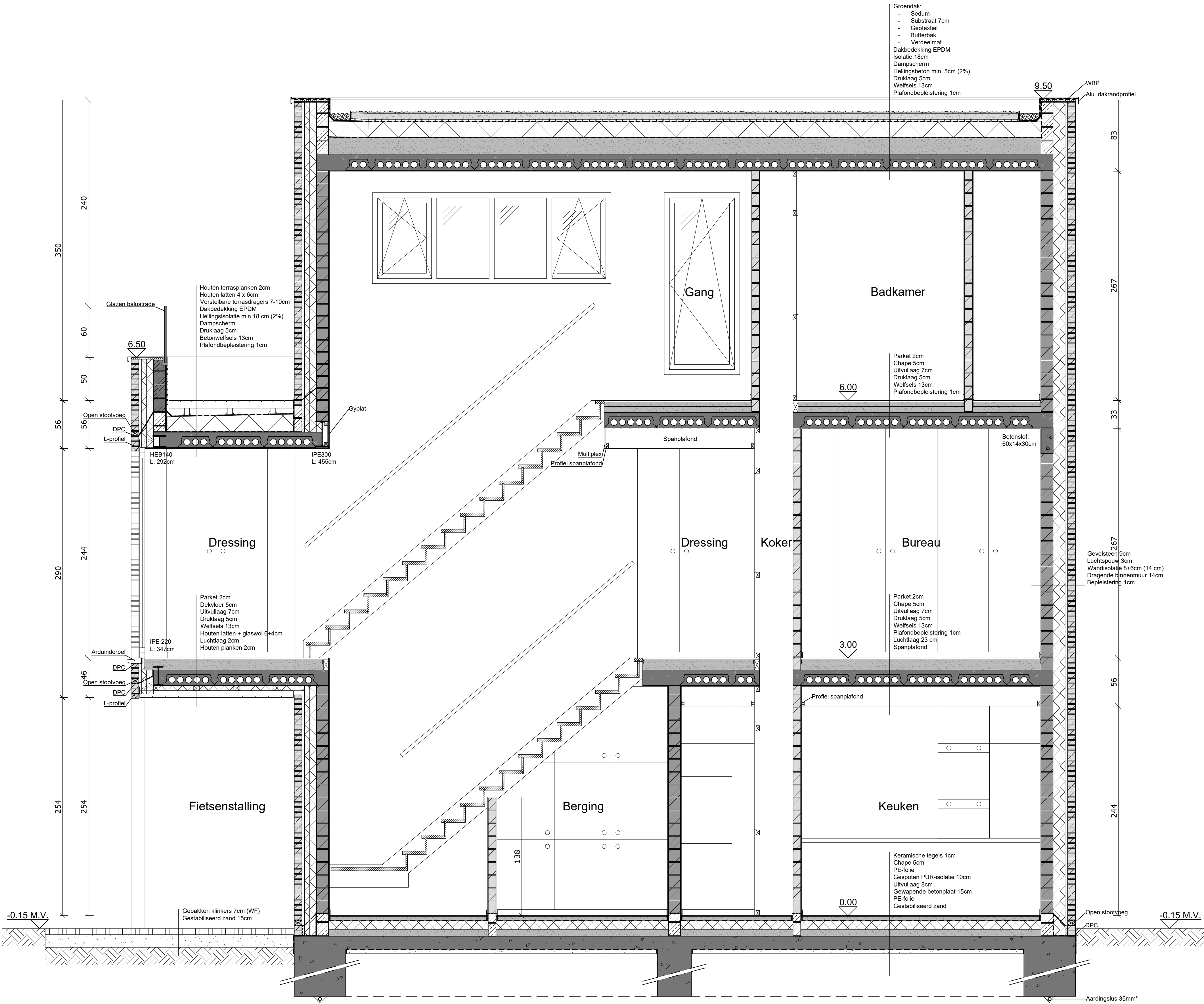
Doorsnede AA'
